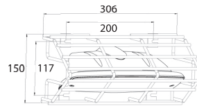
Beschermkorf wandmodel
