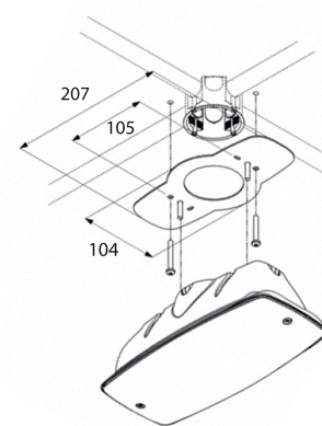
Afdekplaat plafondmodel
